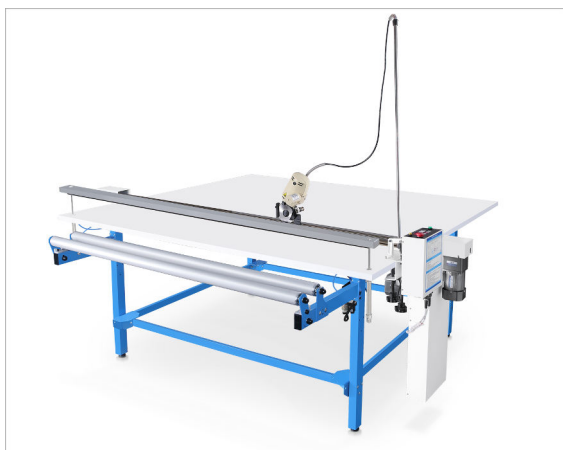
Zestaw z odkrawaczem automatycznym DYDB-2B, odwijakiem rolkowym i pneumatyczną listwą dociskową
