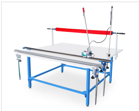
Zestaw z odkrawaczem ręcznym DYDB-1, odwijakiem z jedną rurą i ręczną listwą dociskową
